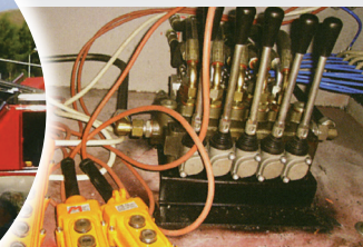
HYDRAULIC PRESS
